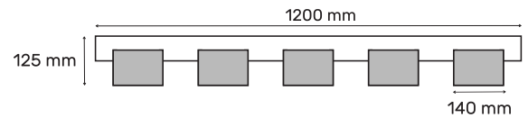
SilentTune_120 A-F / SilentTune_120 B-F 1200 x 1200 x 125 mm
