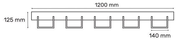
SilentTune_120 A / SilentTune_120 B 1200 x 1200 x 125 mm
