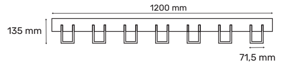
SilentTune_120 A / SilentTune_120 B 1200 x 1200 x 135 mm
